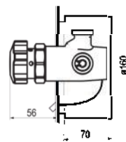
Con válvula de vaciado y conducto guía
