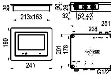
Pantalla + módulo hidráulico
