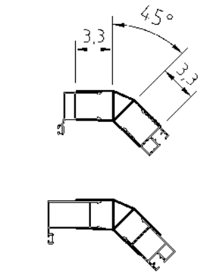
Profilo di congiunzione / Junction profile
