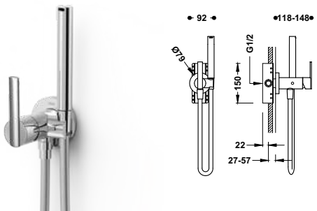
Grifo monomando empotrado con ducha para inodoro Opción para paredes de Pladur. Con agua fría o caliente. Ducha de mano con racor limitador a 5 l/min. y sistema antigoteo. Soporte fijo para la ducha de mano instalable a derecha o izquierda. Flexo satinado.
