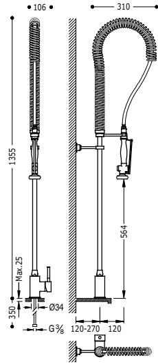
Grifo monomando con ducha extraíble para cocina industrial Con latiguillos de alimentación flexibles G3/8.
