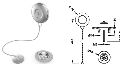
Cazoleta plana de desagüe con kit de enganche de cadenilla y tapón para bañera Cadenilla: 450 mm. Cazoleta: Ø 70 mm. Tapón metálico.
