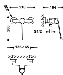
Grifo monomando medical mural para ducha Ducha de mano anticalcárea. Soporte articulado para ducha de mano. Flexo metálico.
