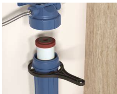
Filtro purificador Seven+: filtra contaminantes y virus, ofreciendo agua más segura y de mejor sabor.
