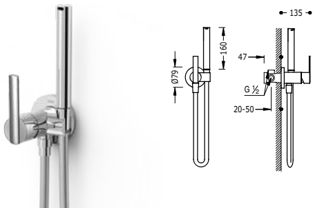
Grifo monomando empotrado con ducha para inodoro Con agua fría y caliente. Ducha de mano con racor limitador a 5 l/min. y sistema antigoteo. Soporte fijo para la ducha de mano instalable a derecha o izquierda. Flexo satinado.
