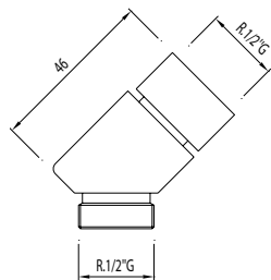
Conexión acodada universal para ducha de mano Apto para bañeras de repisa. Para ref.: 14150, 61150, 62150, 63145, 61161, 87150, 87161, 89150, 89161.
