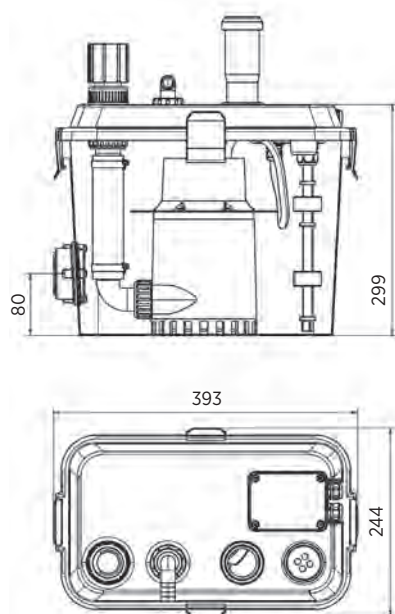
Dimensiones (mm)
