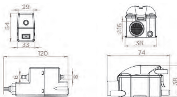
Dimensiones (mm)
