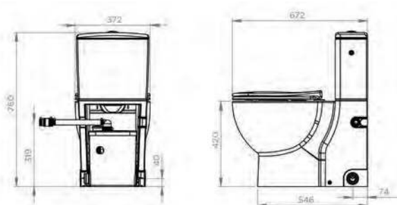
Dimensiones (mm)
